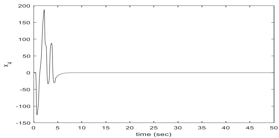
(d) The time response of states x_4
